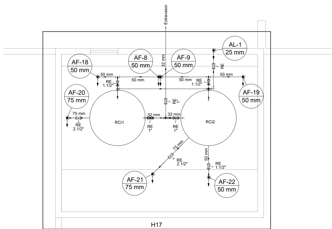
03 PROJETO DA CAIXA D'ÁGUA ESCALA: 1:100
