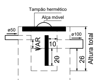
Caixa de gordura Corte 1 - ESC. 1:25
