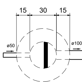
Caixa de gordura Planta baixa - ESC. 1:25
