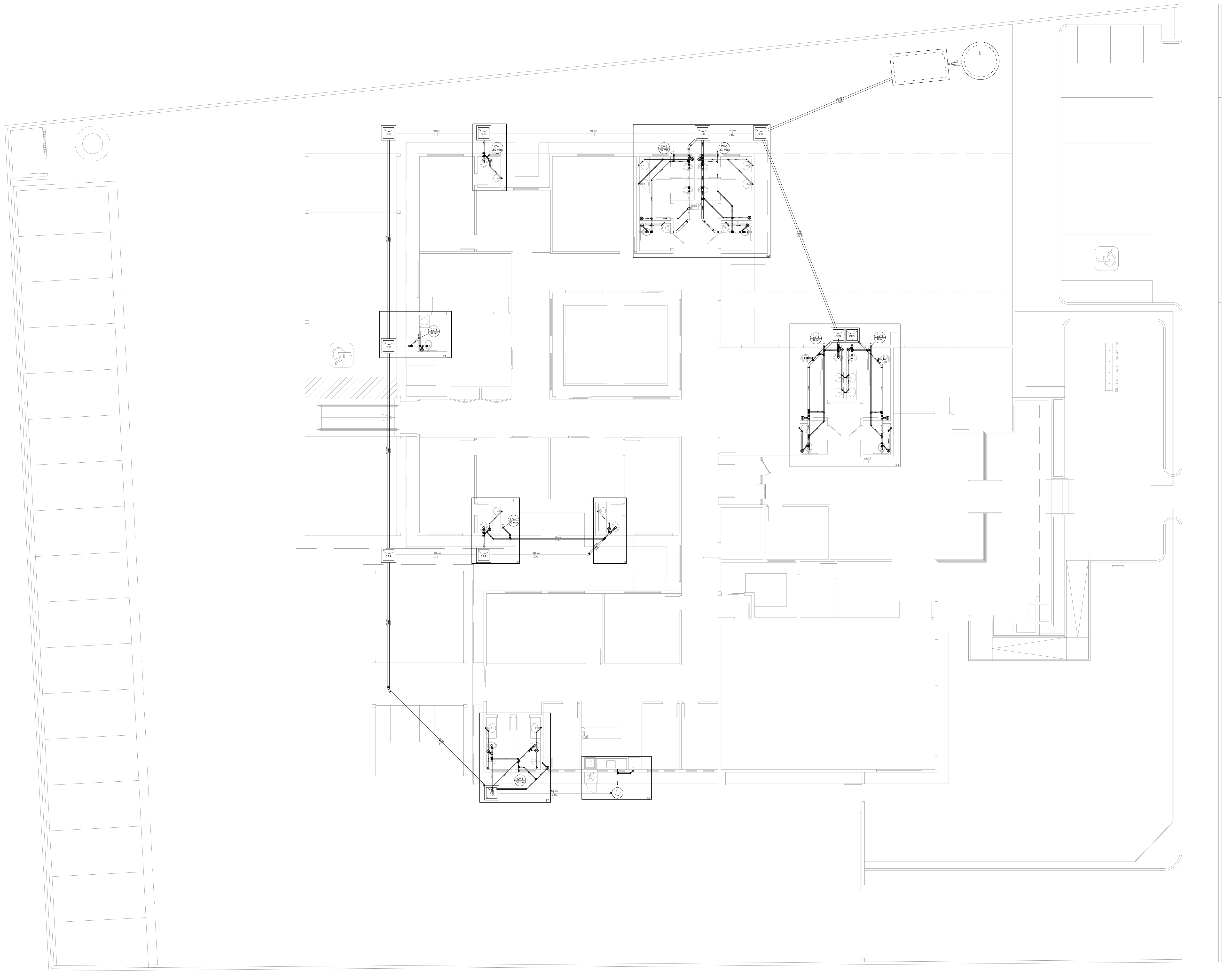
01 PROJETO DO TÉRREO ESCALA: 1:100
