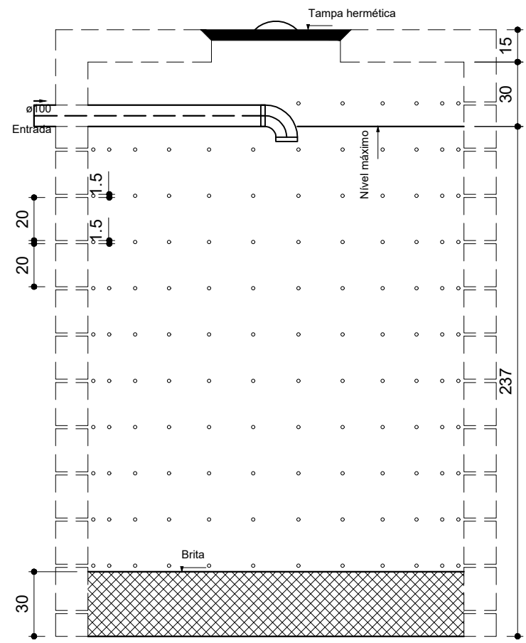
Sumidouro Corte 1 - ESC. 1:25
