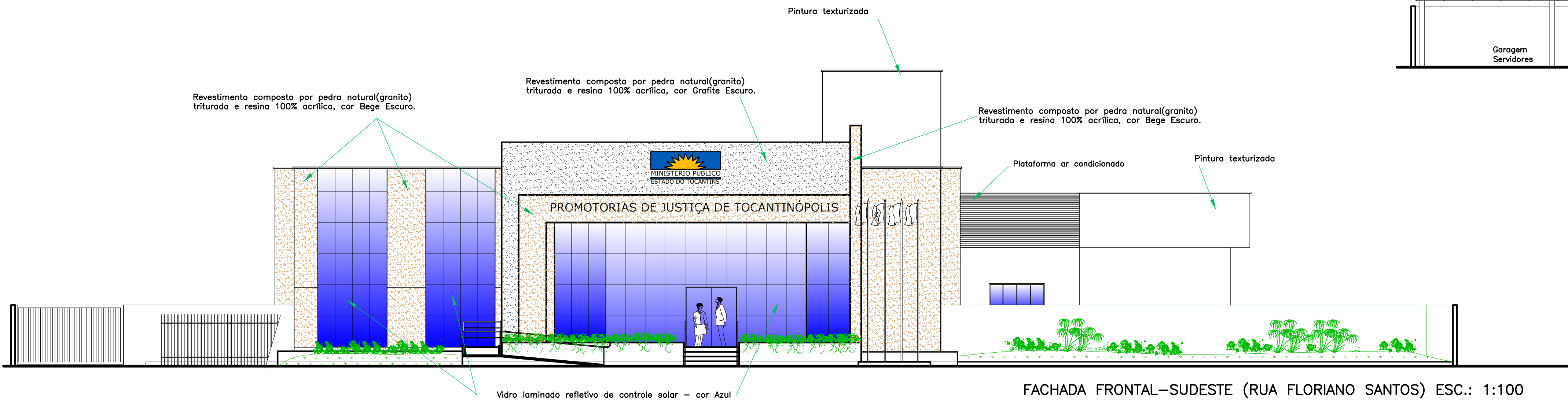
FACHADA FRONTAL-SUDESTE (RUA FLORIANO SANTOS) ESC.: 1:100
