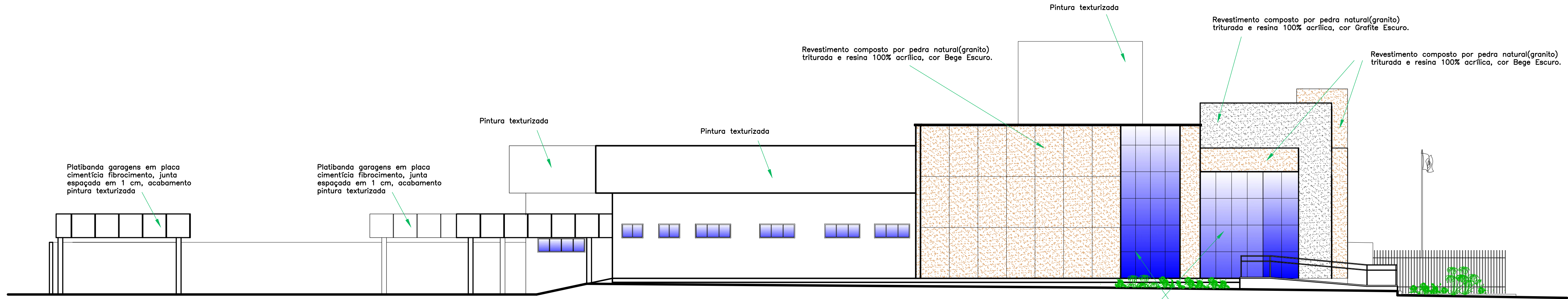
FACHADA LATERAL-SUDOESTE ESC.: 1:100
